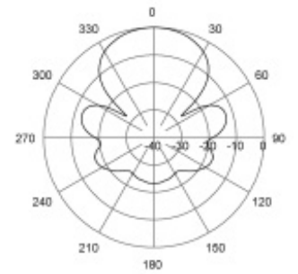
H-Plane | 445 MHz
